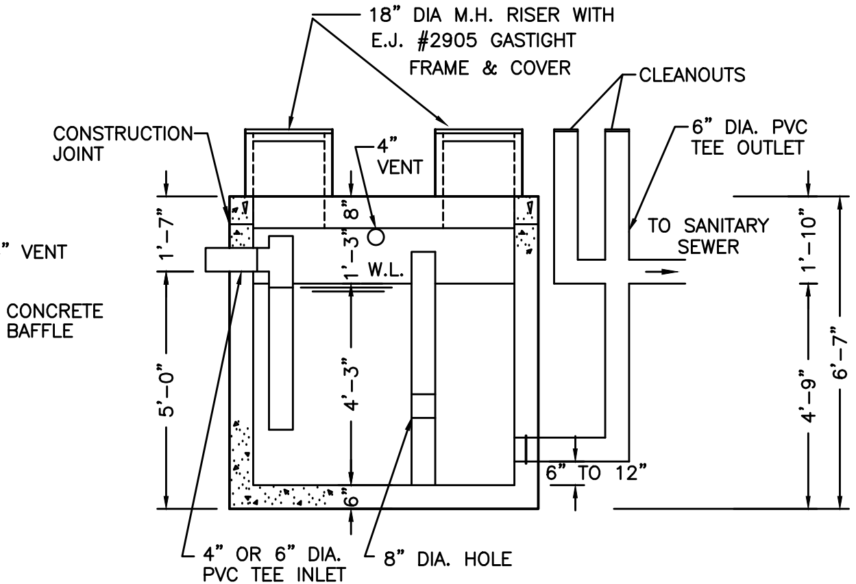
SECTION A-A
